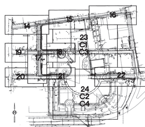
UTILITIES PLAN SHEET INDEX N.T.S.
